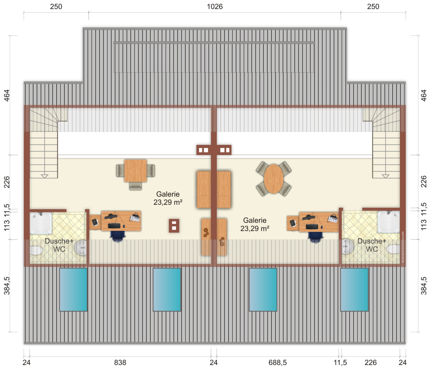
2. Dachgeschoß
