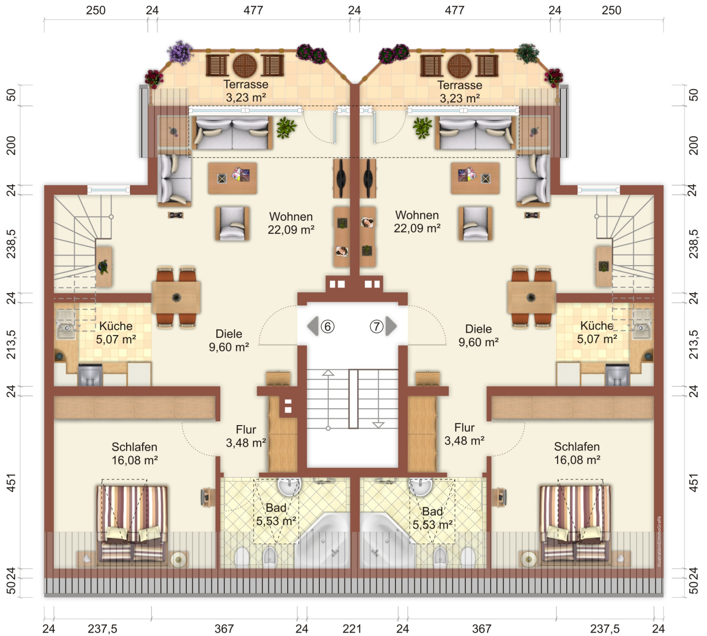
1. Dachgeschoß
